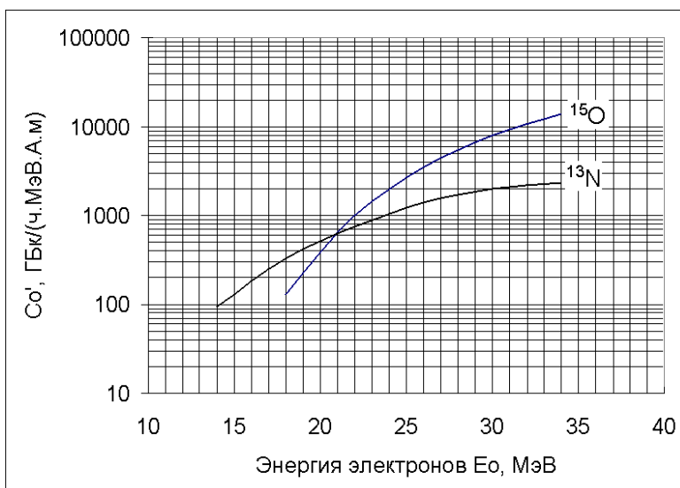
Рисунок 1. Зависимость постоянной скорости образования ( C'_0 ) радионуклидов ^{13}\text{N} и ^{15}\text{O} от энергии электронов (вольфрамовая мишень).
